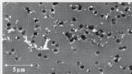
Partikel der realen Umgebungsluft
